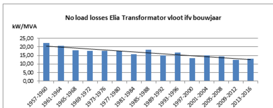
Figuur 3.3: Transformatorverliezen
