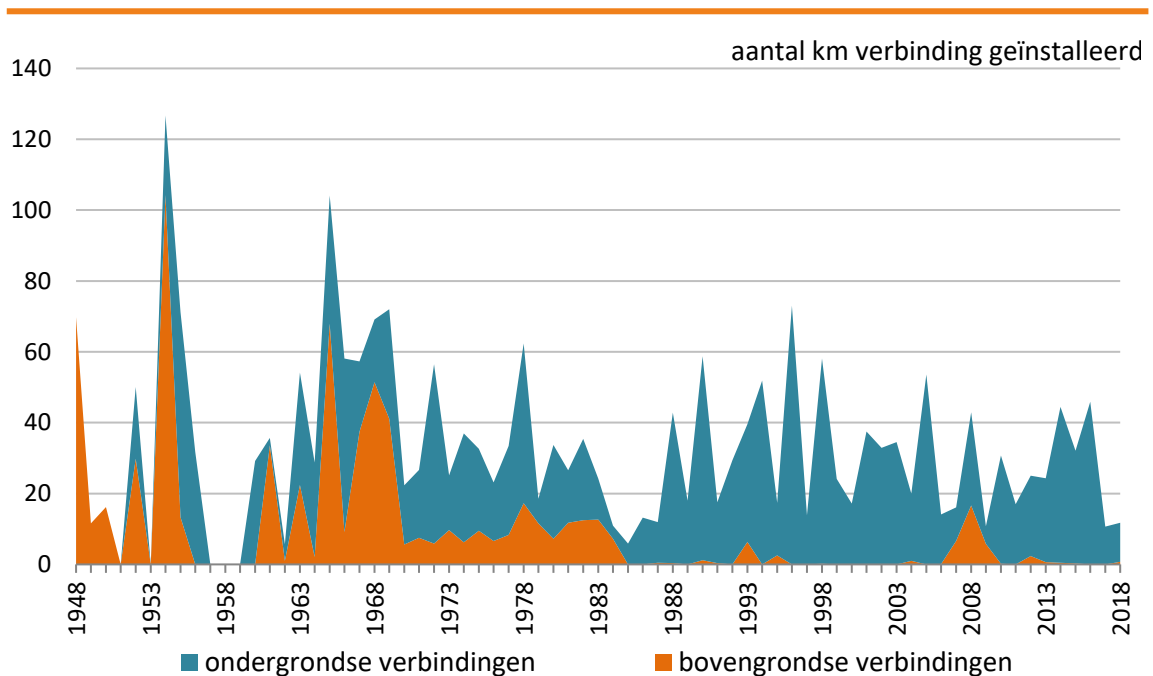
Figuur 2.3: Uitsplitsing van de verbindingen naar bouwjaar
